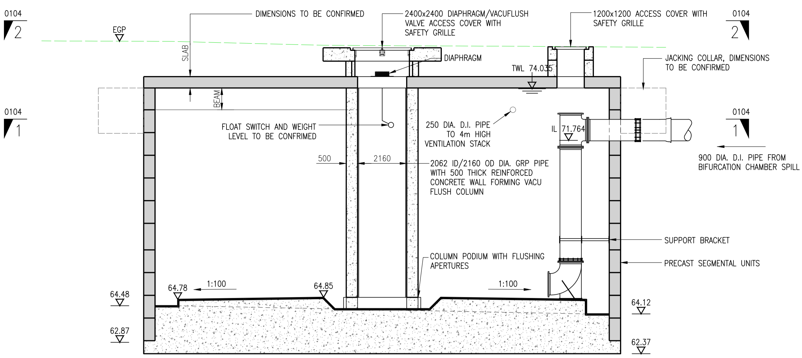
SECTION A-A
